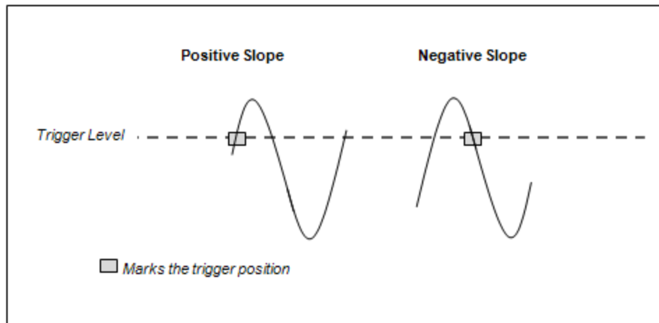
Figure 4-2 Edge Triggers
